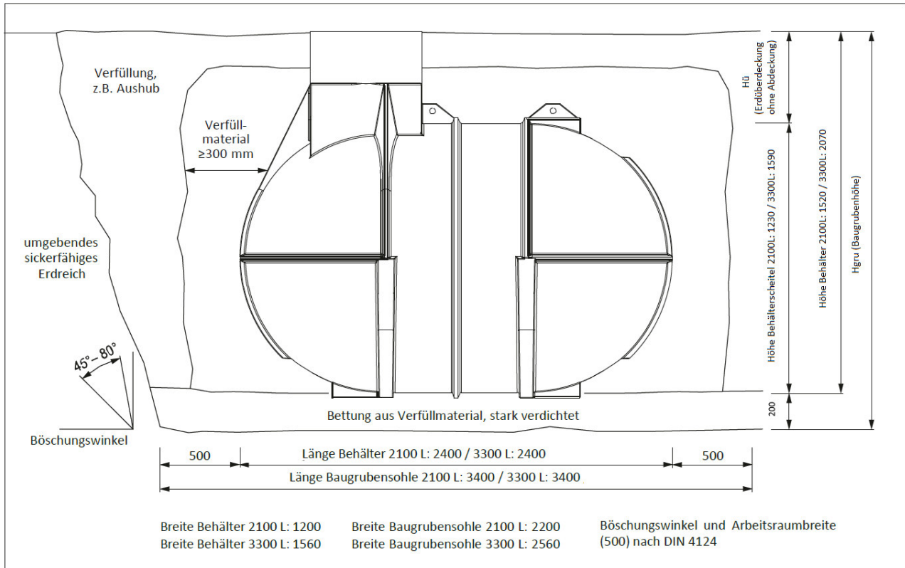
Abbildung 2: Einbaugrößen
