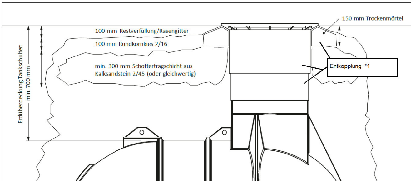
Abbildung 5: Bauseitige Herstellung eines befahrbaren Überbaus mit Teleskopdom
